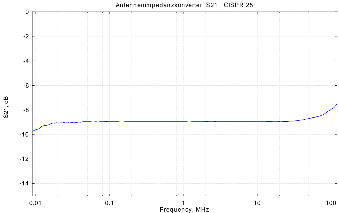
Übertragungsmaß S21 mit Antennennachbildung nach CISPR 25 am Eingang. Transmission with Artificial Antenna Network (CISPR 25) at the Input.
