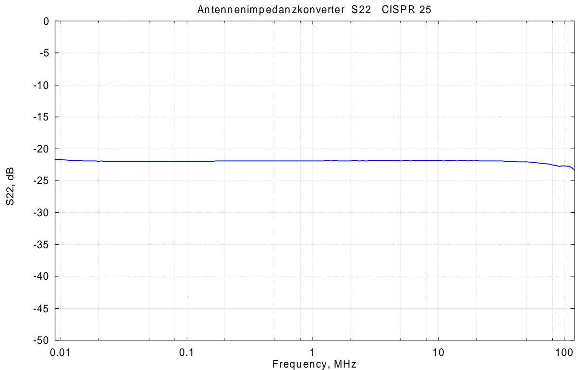
Ausgangs Anpassung S22. Output Return Loss.
