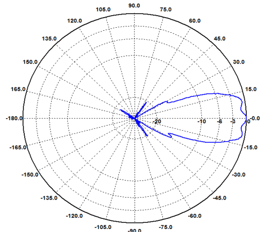
H-Ebene / H-Plane 15 GHz
