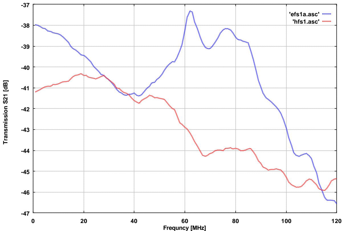
Transmission der Streifenleitung TEMZ 5238 über E-Feldsonde EFS 9218 bzw. H-Feldsonde HFS 1546
