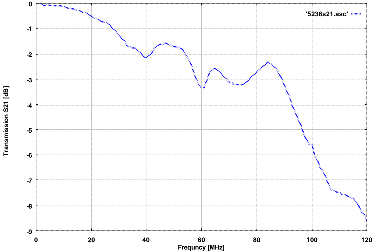
Transmission der Streifenleitung TEMZ 5238 Transmission of the TEMZ 5238 Stripline
